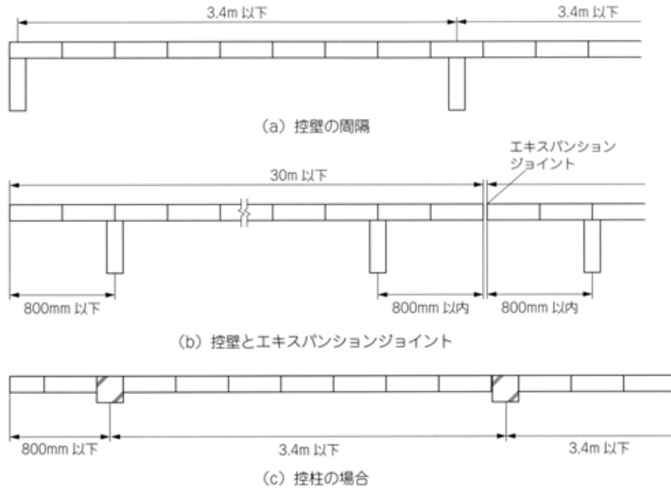
図14-3 控壁・控柱・エキスパンションジョイントの配置
