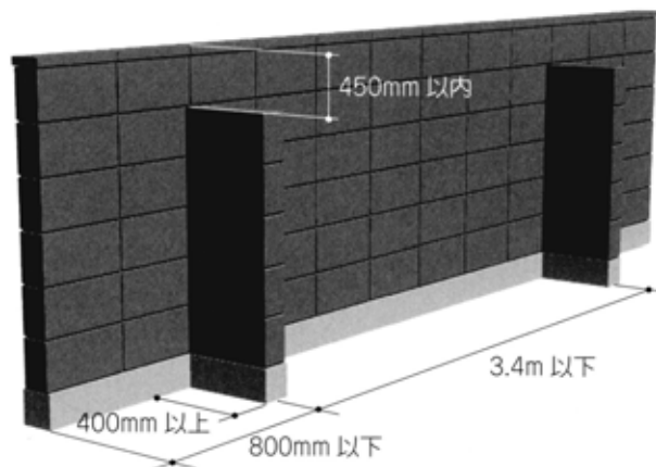
図14-5(b) 控壁の規定
