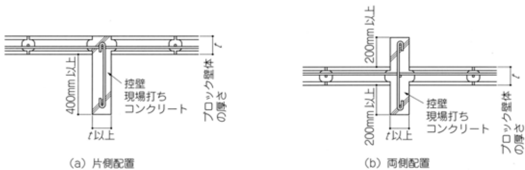
図14-6 RC造控壁の例
