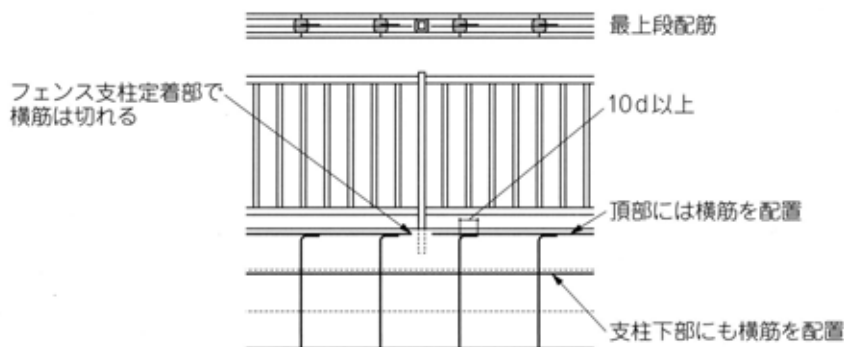
図19-28 フェンス支柱周り
