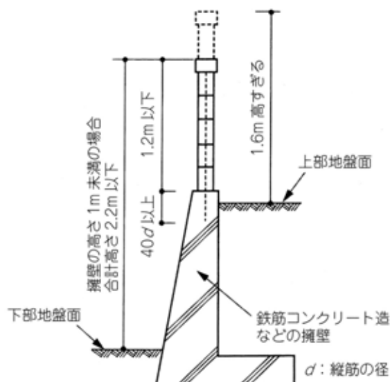
図14-4 擁壁の上部に塀を設ける場合の限度
