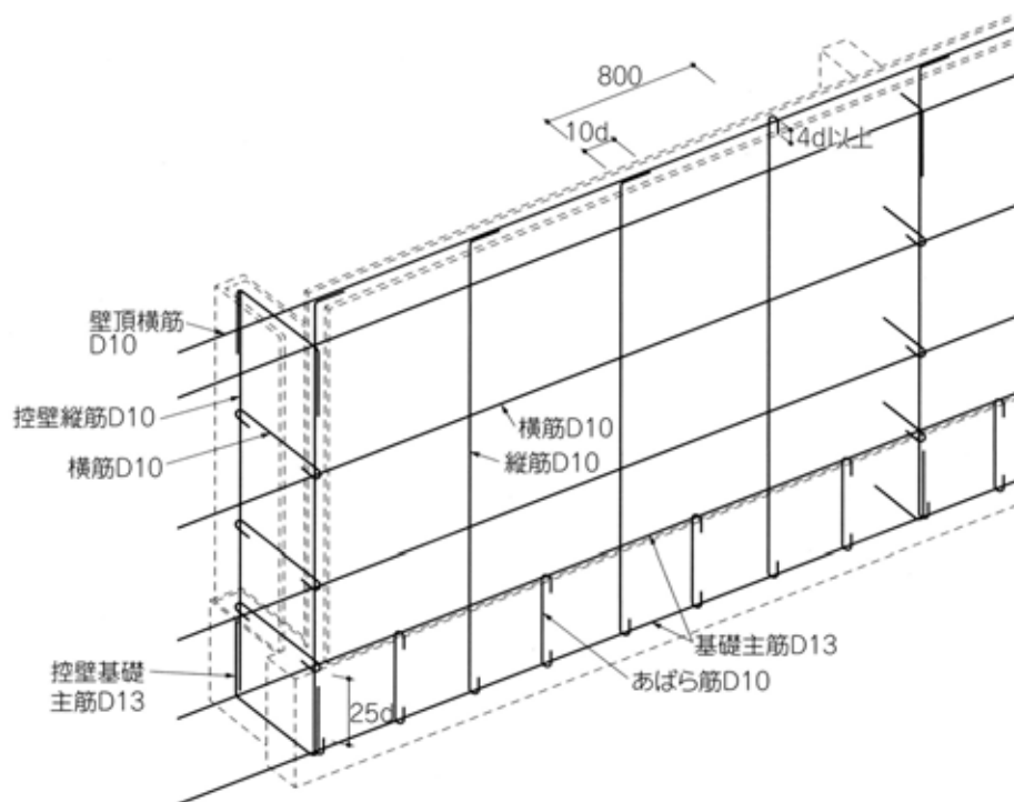
図14-8 ブロック塀の配筋例
