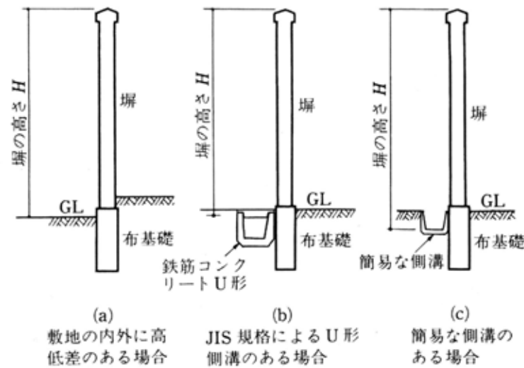
図14-1 塀の高さの測り方
