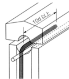
図19-27 かさ木例（えぐりあり）
