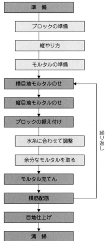
図19-15 ブロックの組積フロー
