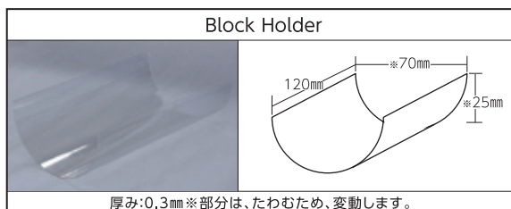
【形状寸法図】
