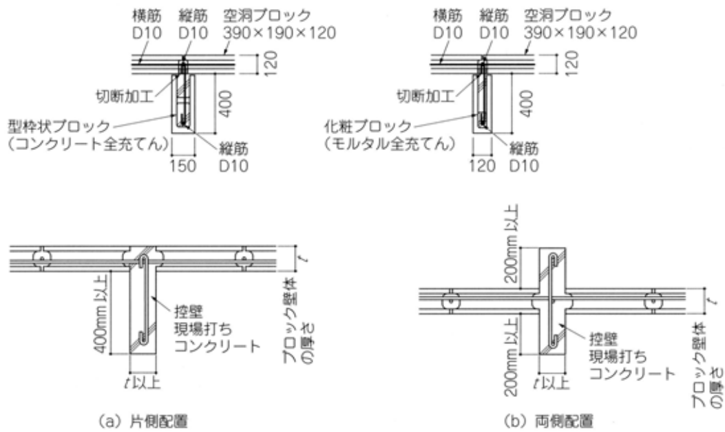
図19-26 控壁の設置例
