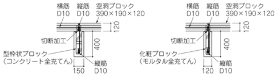
図14-5(a) ブロックを用いた控壁の例
