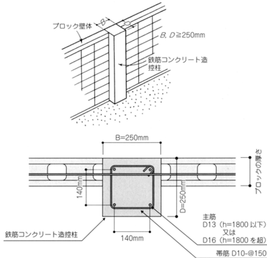
図14-7 控柱の配置例
